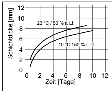
Diagramm 1: Durchhärtageschwindigkeit für Sikaflex®-252i
